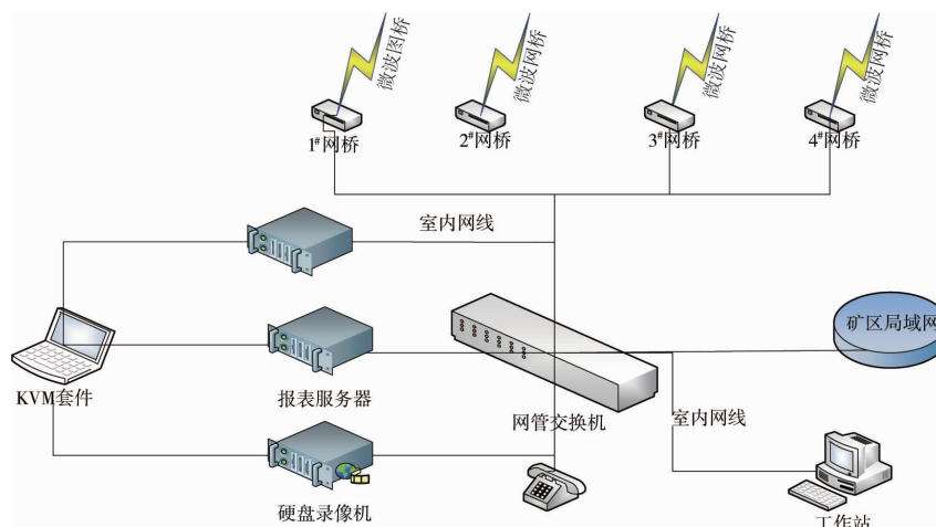
图 2 卡调系统工作网络
