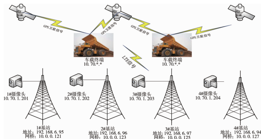
图 1 卡调系统构架
